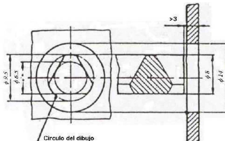
Fig. 4.- Triángulo de desenclavamiento (cotas en milímetros)
